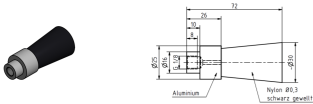
Pinsel Ø30 mit Halterung und Steckanschluss gerade Bestellnr.: 10100668 Zeichnungsnr.: AZ300012
