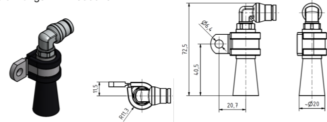
Pinsel Ø20 mit Haltewinkel Bestellnr.: 10100672 Zeichnungsnr.: AZ300016
