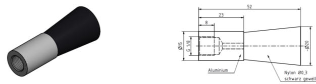
Pinsel Ø20 mit Halterung und Steckanschluss 90° Bestellnr.: 10100669 Zeichnungsnr.: AZ300013
